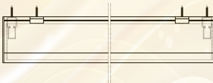
bevestiging kast door ophangprofiel fixation de caisson par profil de suspension
